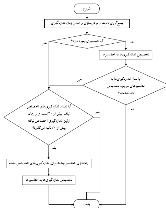
شکل ۴: فلو چارت فرایند واسته‌سازی داده
