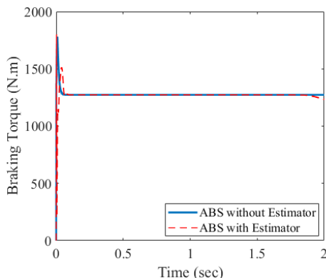
شکل ۱۴: مقایسه گشتاور کنترلی با و بدون تخمین‌زن
