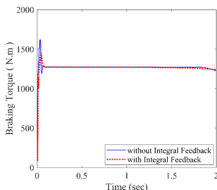
شکل ۱۸: مقایسه گشتاور کنترلی، کنترل‌کننده با فیدبک انتگرال و بدون فیدبک انتگرال
