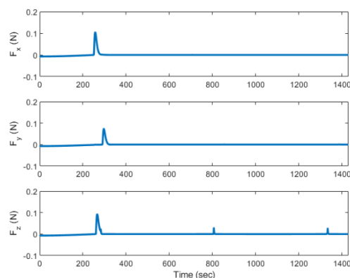
شکل ۹: نیروی کنترلی اعمالی جهت نگهداری ماهواره بر روی مدار مرجع در روش کنترل پیش‌بین
