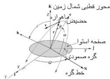
شکل ۳: تعابیر فیزیکی المان‌های مداری [۱۵]
