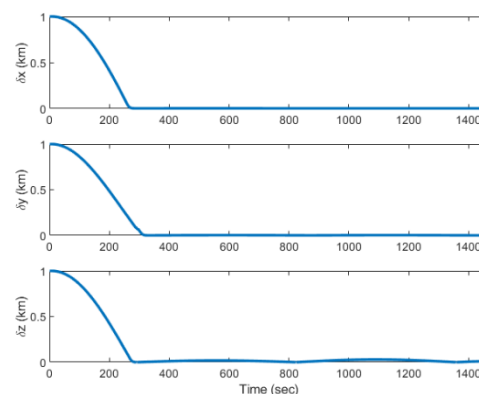
شکل ۸: خطای بین مدار مرجع و ماهواره در روش کنترل پیش‌بین
