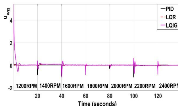
شکل ۱۴: مقایسه سیگنال کنترل‌کننده‌های PID، LQR و LQIG
