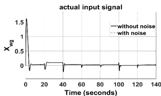
شکل ۲۳: باز شدن واقعی دریچه برای مدل غیرخطی با و بدون نویز
