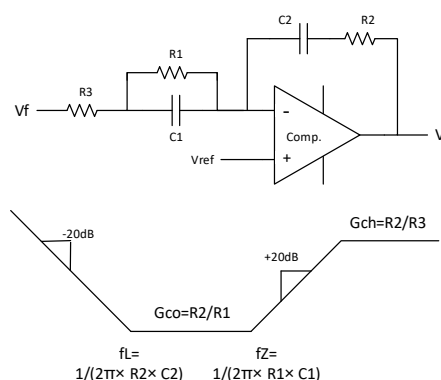
شکل ۱۳: جبران ساز
