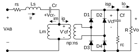
شکل ۲: متغیرهای حالت در مبدل رزناسی سری
