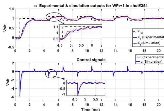
شکل ۱۶: مقایسه پاسخ مدل M1_{10} برای نقطه کار +۱ در شرایط واقعی با شات ۳۵۴. a- خروجی واقعی دستگاه و خروجی مدل b- سیگنال های کنترلی شبیه سازی و عملی.
