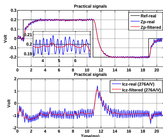
شکل ۶: حذف دینامیک‌های سریع ناشی از بلوک هیستریزس از سیگنال‌های
