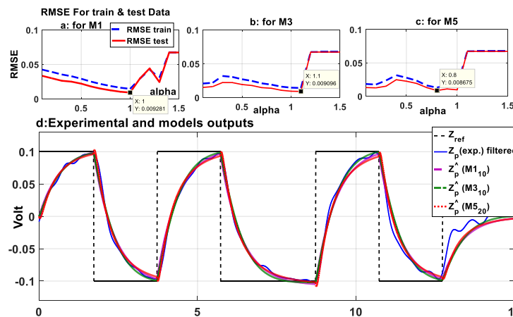
شکل ۱۲: a- خطای RMSE بر حسب \alpha برای ساختار مدل M1، b- خطای RMSE بر حسب \alpha برای ساختار مدل M3، c- خطای RMSE بر حسب \alpha برای ساختار مدل M5، d- مقایسه خروجی عملی و خروجی مدل‌های انتخاب شده برای نقطه کار +۱ در شات تست (#۳۵۴) جدول ۶: نتایج مدل‌های بهینه در نمونه برداریها، ساختارهای مختلف، با معیار خطا برای نقطه کار +۱
