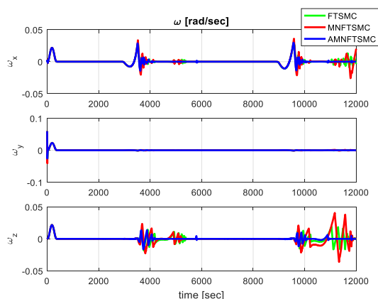
شکل ۲: سرعت‌های زاویه‌ای نانوماهواره برای قانون کنترلی پیشنهادی، FTSMC و MNFTSMC [۱۳]
