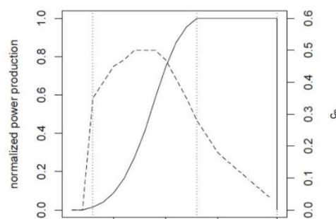
شکل ۷: نمونه‌ای از منحنی توان یک توربین بادی
