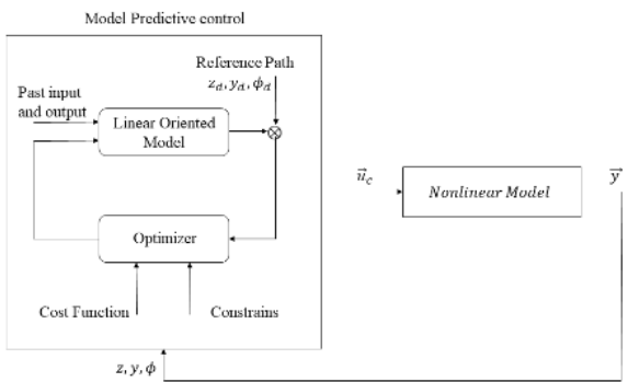
شکل ۷ روند نمای کنترل پیش بین مبتنی بر مدل طراحی شده تابع هزینه و قیود
