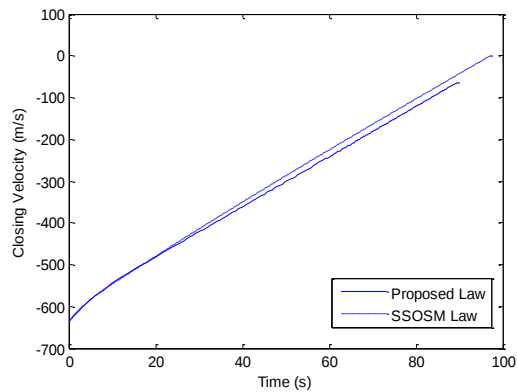
شکل ۱۶: سرعت نزدیک شونده به رهگیر به هدف در سناریوی درگیری دوم
