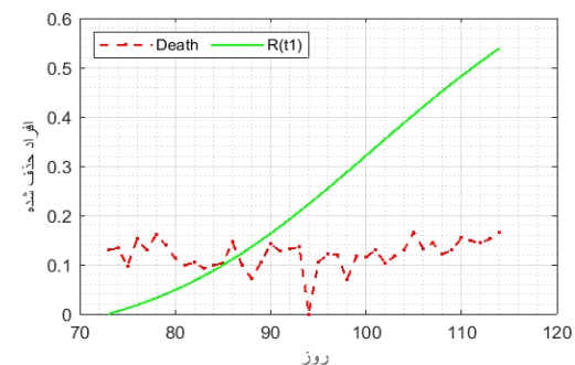
شکل ۳. (الف) نمودار مقایسه افراد مبتلا شده در بازه دوم و تخمین مدل از افراد مبتلا ( a = 0/17 و b = 0/082 ). (ب) نقاط قرمز رنگ تعداد افراد فوت‌شده در اثر کرونا و خط سبز رنگ تخمین مدل از افراد حذف‌شده در بازه دوم.
