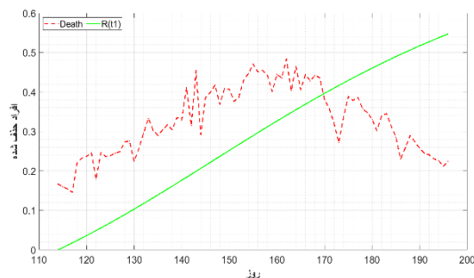
شکل ۴. آ (الف) نمودار مقایسه افراد مبتلا شده در بازه سوم و تخمین مدل از افراد مبتلا ( a = 0/036 و b = 0/063 ). (ب) نقاط قرمز رنگ تعداد افراد فوت‌شده در اثر کرونا و خط سبز رنگ تخمین مدل از افراد حذف‌شده در بازه سوم.
