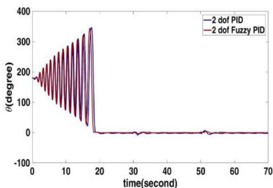
شکل ۹: عملکرد کنترل کننده ها در پایداری سازی زاویه آونگ (swing up به همراه اغتشاشات خارجی)
