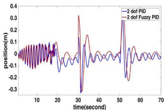
شکل ۸: عملکرد کنترل کننده ها در پایداری سازی موقعیت ارایه (swing up به همراه اغتشاشات خارجی)
