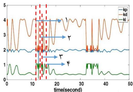
شکل ۱۱: ضرایب کنترل کننده های خود تنظیم فازی PID با دو درجه آزادی در حضور اغتشاشات خارجی
