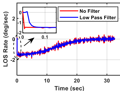
شکل ۱۶: تاثیر فیلتر بر سیگنال تخمین نویز آلود
