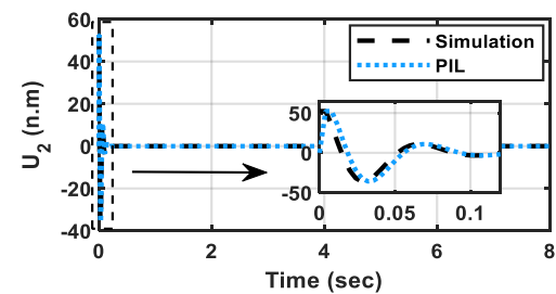
شکل ۱۴- سیگنال‌های کنترل
