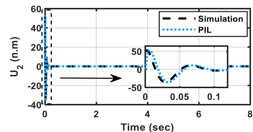
شکل ۱۴- سیگنال‌های کنترل
