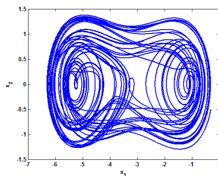
شکل ۳: رفتار آشوبناک سیستم پاندول آشوبناک (صفحه فاز)
