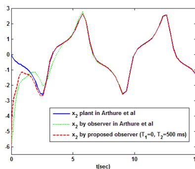
شکل ۷: مسیر حالت سیستم و اندرل، نتایج مقایسه ای روتگر پیشنهادی و روتگر ارائه شده در [۳۵] (Arthure et al)
