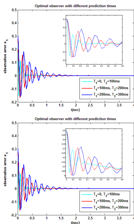
شکل ۵: خطای تخمین حالت سیستم پاندول آشوبناک توسط رویکرد بهینه پیشنهادی به ازای زمان‌های پیش‌بینی مختلف
