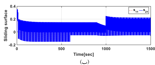
شکل ۷. سطح لغزش (آ) کنترل‌کننده DDASMC پیشنهادی، (ب) کنترل‌کننده MFASMC در مرجع [۵]
