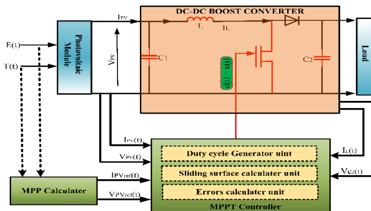
شکل ۶. تصویر مفهومی از عملکرد ساختار کنترلی حلقه‌بسته سیستم فتوولتایی
