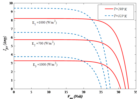
شکل ۳. منحنی مشخصه‌ی جریان I_{pv} بر حسب ولتاژ V_{pv} ماژول فتوولتائی به ازای سه تابش متفاوت E_1 = 1000 \left(\frac{W}{m^2}\right) , E_2 = 700 \left(\frac{W}{m^2}\right) , E_3 = 400 \left(\frac{W}{m^2}\right) و دو دمای مختلف T_1 = 298^\circ K و T_2 = 298^\circ K [۱۵]
