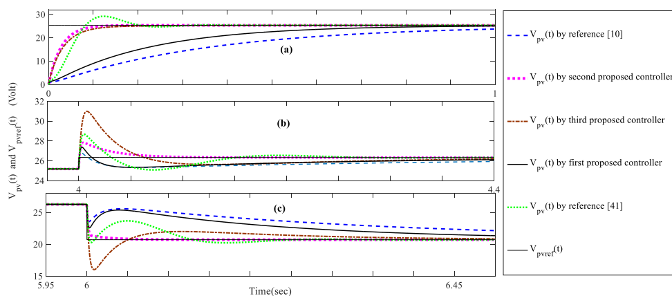
شکل ۹. بزرگنمایی پاسخ زمانی ولتاژ مازول فتوولتائی V_{pv}(t) برای هر پنج راهکار کنترلی، (a): بزرگنمایی پاسخ زمانی V_{pv}(t) در لحظه‌ی \{t_0 = 0\} ; (b): بزرگنمایی پاسخ زمانی V_{pv}(t) در لحظه‌ی \{t_1 = 4\} ; (c): بزرگنمایی پاسخ زمانی V_{pv}(t) در لحظه‌ی \{t_2 = 6\} .
