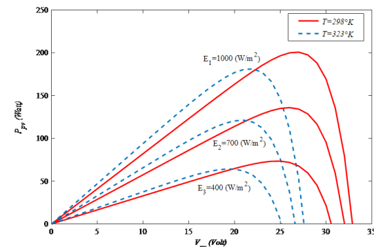
شکل ۴. منحنی مشخصه‌ی توان خروجی P_{pv} لفظه‌ای V_{pv} بر حسب ولتاژ V_{pv} ماژول فتوولتائی به ازای سه تابش متفاوت E_1 = 1000 \left(\frac{W}{m^2}\right) , E_2 = 700 \left(\frac{W}{m^2}\right) , E_3 = 400 \left(\frac{W}{m^2}\right) و دو دمای مختلف T_1 = 298^\circ K و T_2 = 298^\circ K [۱۵]
