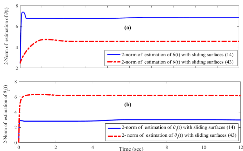
شکل ۵. پاسخ‌های زمانی نرم اقلیدسی بردارهای تخمینی \|\theta(t)\| و \|\theta_f(t)\| : (a) پاسخ‌های زمانی \|\theta(t)\| با وجود سطوح لغزشی (۱۴) و (۴۳); (b) پاسخ‌های زمانی \|\theta_f(t)\| با وجود سطوح لغزشی (۱۴) و (۴۳)
