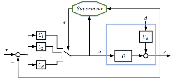
شکل ۱- ساختار کلی کنترل نظارتی کلیدزن
