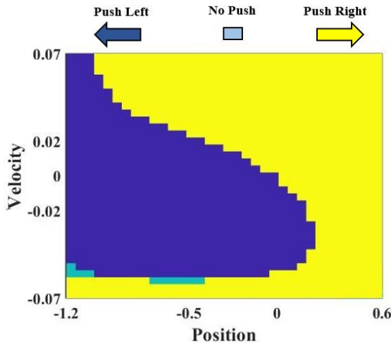
شکل ۹: سیاست یادگرفته شده توسط NLSPI بر روی کل فضای ورودی
