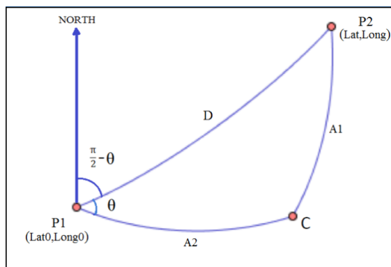
شکل ۷- تصویر مسیر حرکت روی کمان های طول و عرض جغرافیایی [۸و۶]
