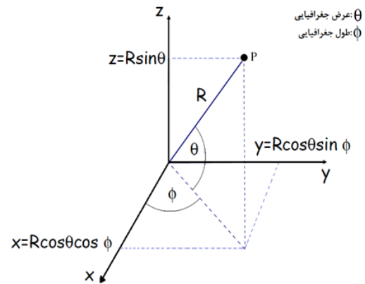
شکل ۵- مولفه های موقعیت در دستگاه کروی [۸و۶]
