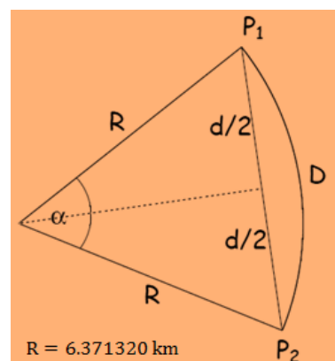
شکل ۶- محاسبه قطاع کره با استفاده از قانون کسینوس و مثلث متساوی الساقین [۸و۶]
