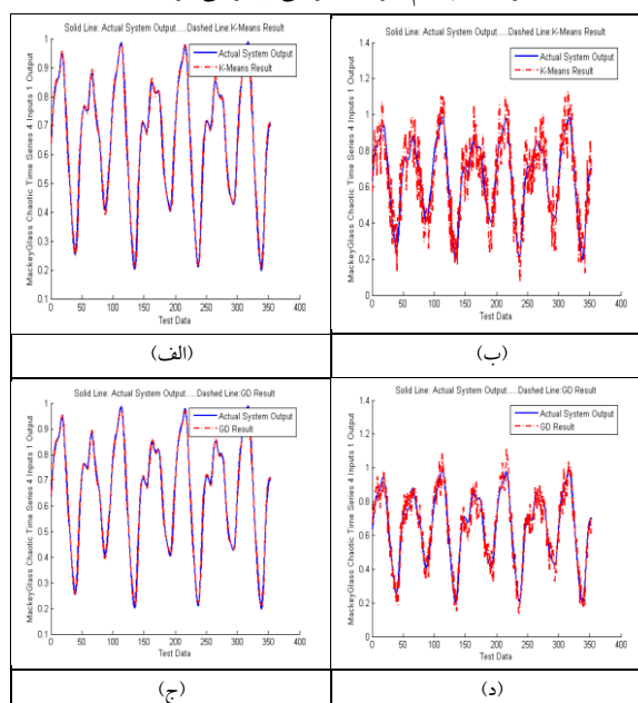
شکل ۷. پیش‌بینی سری زمانی مکی گلاس توسط شبکه عصبی RBF گرانولی با ۲۰ ترون لایه میانی و به روش (الف) «الگوریتم خوشه‌بندی K-Means» و بدون نویز (ب) «الگوریتم خوشه‌بندی K-Means» و SNR=0 (ج) «الگوریتم گرایان نزولی» و بدون نویز (د) «الگوریتم گرایان نزولی» و SNR=0
