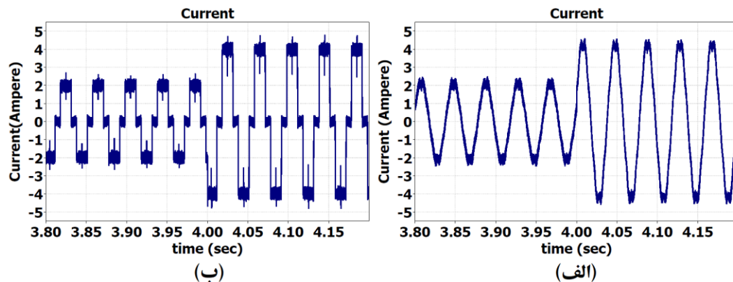
شکل ۲۴- جریان فاز موتور BLDC با روش‌های الف) DP-FCS-MPC و ب) CC-FCS-MPC در سرعت ۱۵۰۰ RPM و تغییر گشتاور 0.1 \text{ N.m} تا 0.2 \text{ N.m} در زمان ۴ ثانیه
