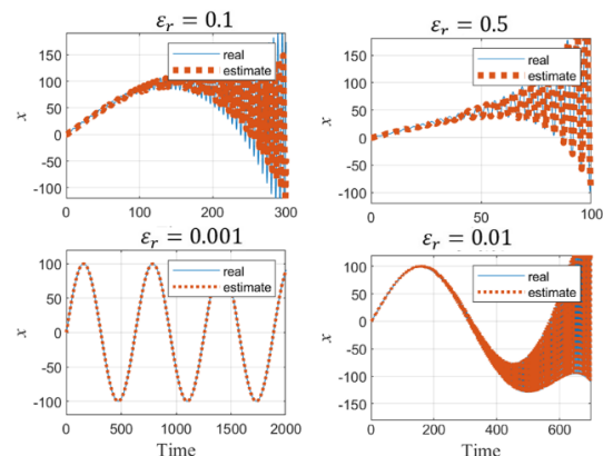
شکل ۳: بررسی اثر انتخاب مقادیر مختلف \varepsilon_r بر تخمین موقعیت رهبر در راستای محور x در سیستم حلقه بسته.
