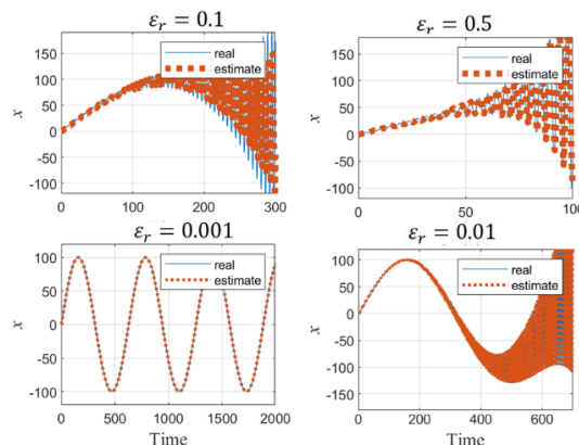
شکل ۱: بررسی اثر انتخاب مقادیر مختلف \varepsilon_r بر تخمین موقعیت رهبر در راستای محور x در سیستم حلقه بسته.
