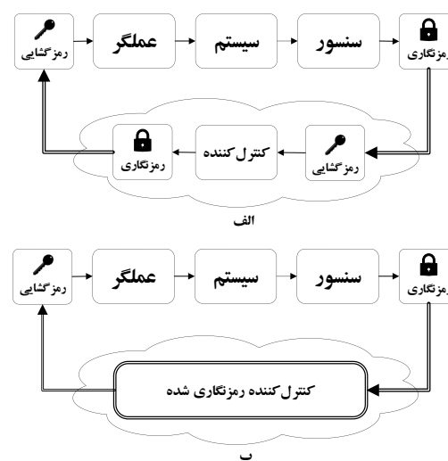
شکل ۲. کنترل کننده مستقر در فضای ابری با کانال های مخابراتی امن (الف) در مقایسه با روش کنترل رمزنگاری شده (ب).
